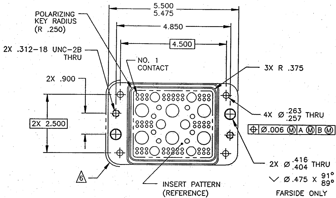
VIEW A-A (-1)
