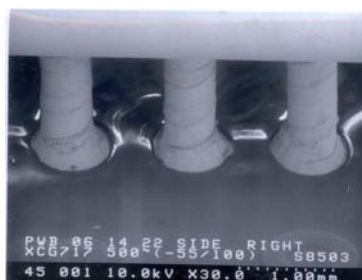
SEM 500 Thermal Cycles (-55/100°C)
