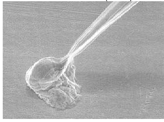
F. Thinning of a whisker (x2200)
